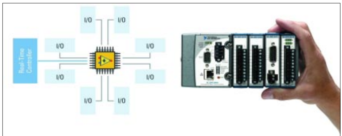
Figure 1. Sistema embebido CompactRIO basado en FPGA
