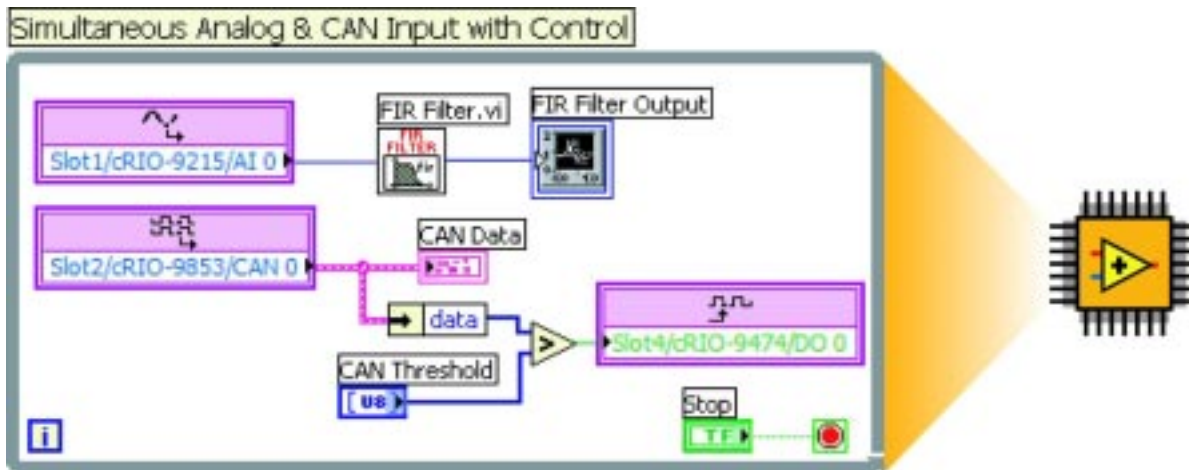
Figura 2. Programación gráfica para FPGAs con LabVIEW
